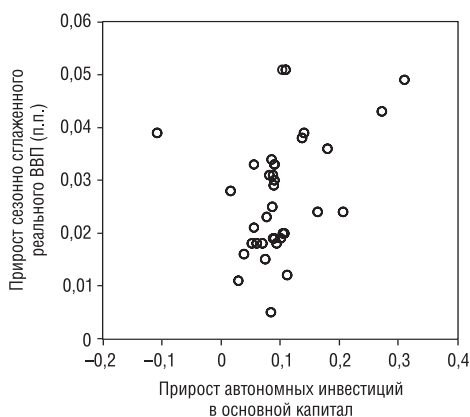
Рис. 6. Диаграмма рассеяния: прирост сезонно сглаженного реального ВВП и прирост автономных инвестиций в основной капитал в ценах I квартала 1999 года, I кв. 1999 — IV кв. 2007 года
