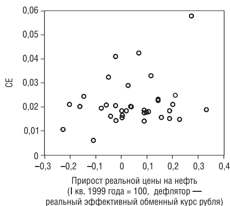
Рис. 9. Диаграмма рассеяния: прирост реальной цены на нефть и остатки коинтеграционного соотношения между приростом ВВП, уровнем цены на нефть и приростом автономных инвестиций, I кв. 1999 — IV кв. 2007 года
