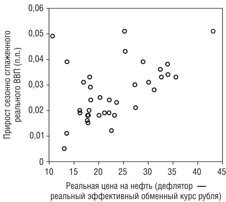
Рис. 4. Диаграмма рассеяния: прирост сезонно сглаженного реального ВВП и реальная цена на нефть в ценах I квартала 1999 года, I кв. 1999 — IV кв. 2007 года
